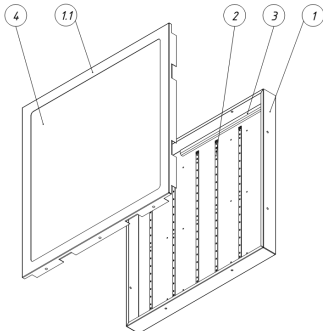
Рисунок 2 - Состав светильника Geniled Office Clip-In.
